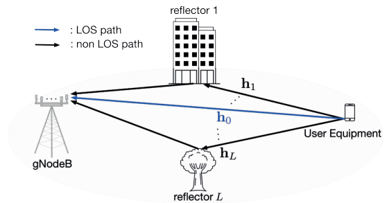
그림 1. 5G NR 프리앰블 기반 OFDM-ISAC 시스템 모델
